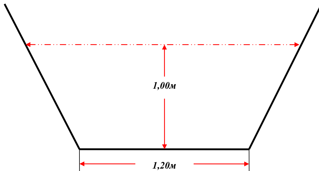
Прилог бр. 10. Карактеристичан попречни профил корита одводног канала-путног канала у КО Велика Биљаница
