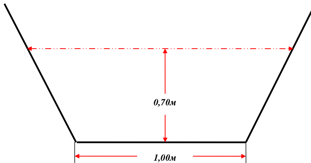
Прилог бр.13. карактеристични попречни профил корита канализа. „Бучило“ у КО Д. Бријање од асфалтног пута према Пустој реци
