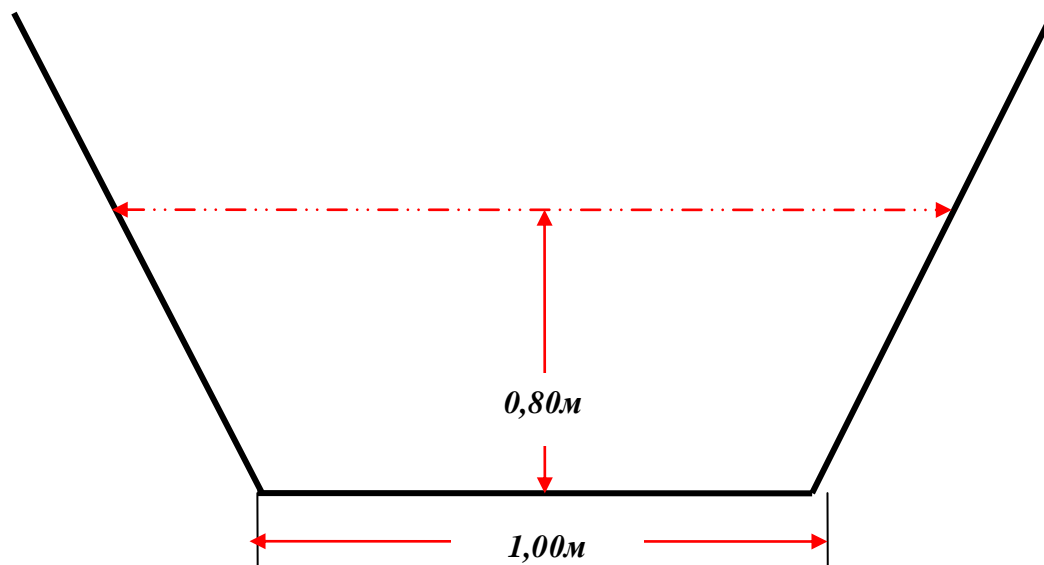
Прилог бр. 3.а – Карактеристичан попречни профил корита канала „Пргон“ у КО Залужње-измуљавање
