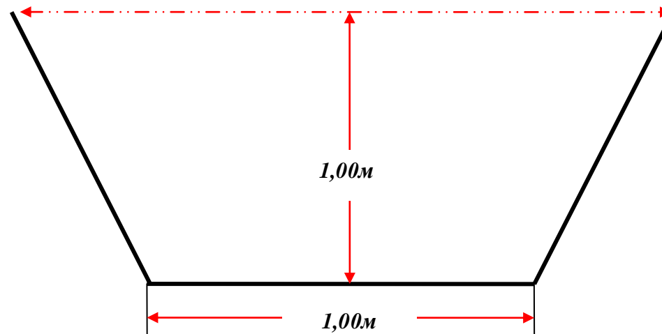
Прилог бр. 3.б. – Карактеристичан попречни профил корита“Пргон“ у КО Залужње–ископ новог корита
