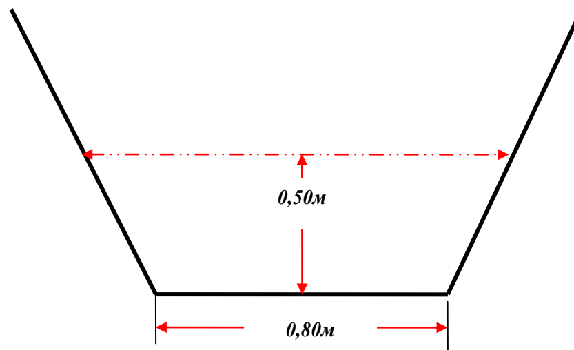
Прилог Бр.12. карактеристичан попречни профил корита путног одводног канала у КО Горње Трњане
