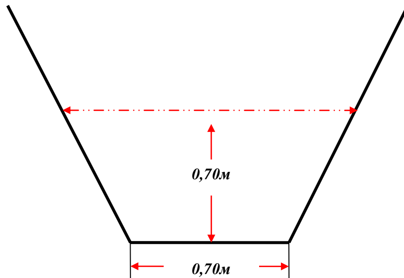
бр. 2 – Карактеристичан попречни профил корита канала КО Доња Локошница
