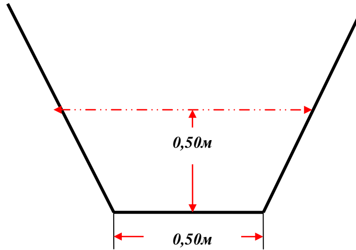
Карактеристичан попречни профил корита одводног канала у КО Мирошевце
